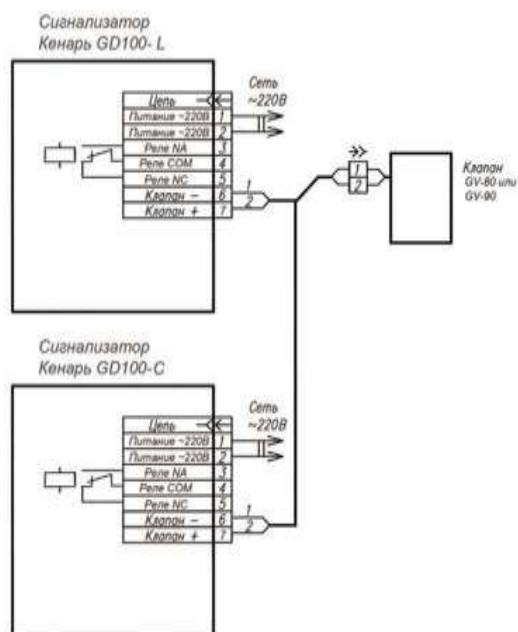
Схема соединения приборов
