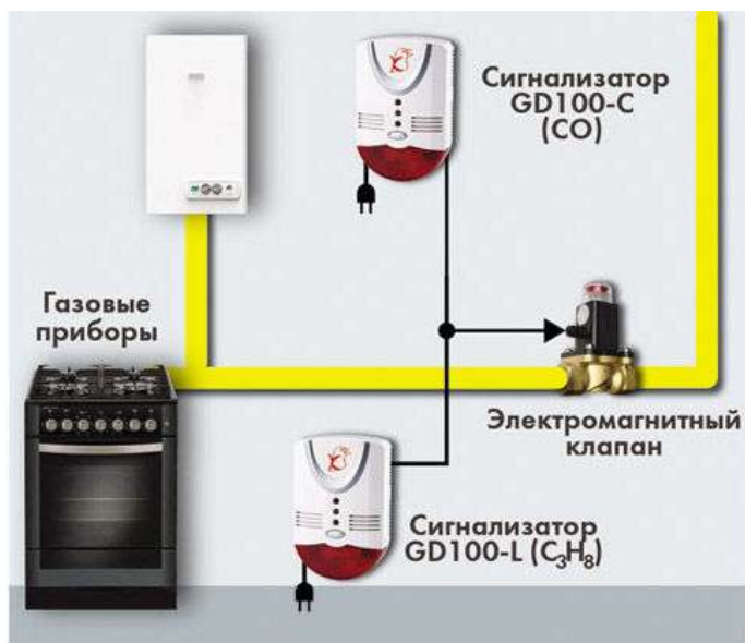
Пример размещения оборудования
